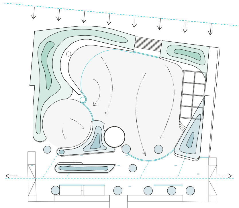
Diagrama de la gestió de les aigües d'escorrentia
